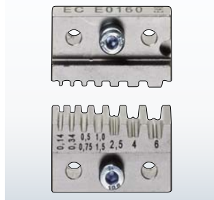
Матрицы для CF 500
