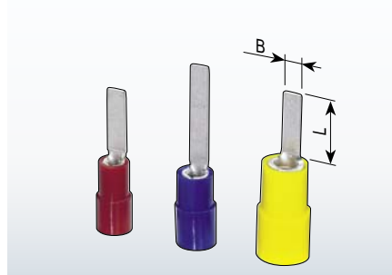
Плоские кабельные наконечники прямые изолированные
