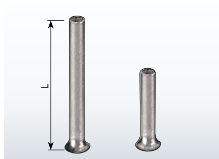
Кабельные наконечники без изоляционных втулок согласно DIN 46228-1
