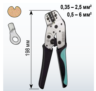
CRIMPFOX-RC 2,5 1212063
