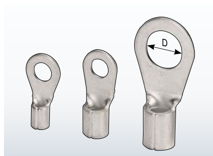
Кольцевые кабельные наконечники неизолированные (продолжение)
