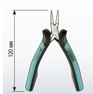
MICROFOX-F плоскогубцы 1212493
