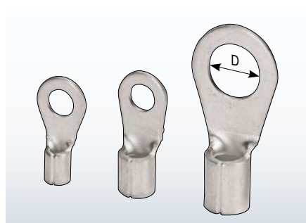
Кольцевые кабельные наконечники неизолированные
