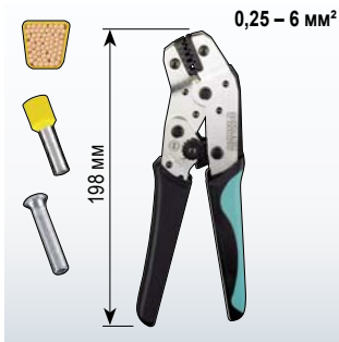
CRIMPFOX 6 1212034
