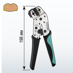
CRIMPFOX-DSUB 5 HD 1212111 CRIMPFOX-DSUB 5-1 Stand. 1212711 Инструмент для опрессовки катаных контактов D-SUB High-Density/Standart, 0,08 мм² - 0,5 мм²
