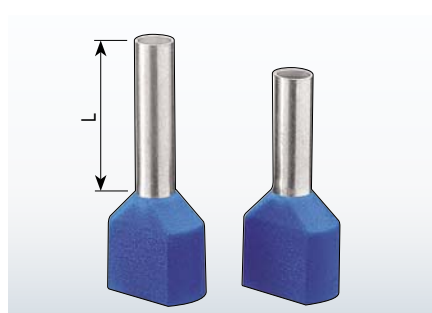
Кабельные наконечники для обжатия двух проводов одним наконечником
