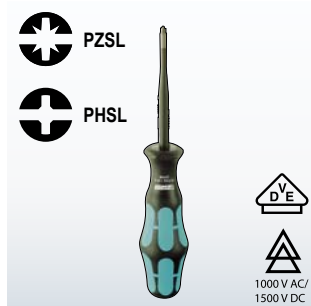
Отвёртки VDE Phillips-Recess®
