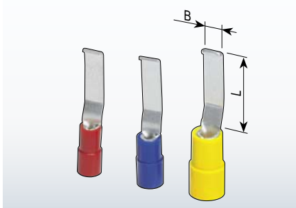
Плоские кабельные наконечники с крючком изолированные
