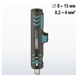
WIREFOX-D 13 1212162
