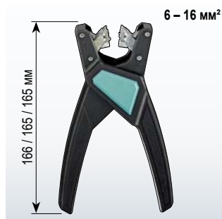
WIREFOX 16-1 6 – 16 мм² 1212157
